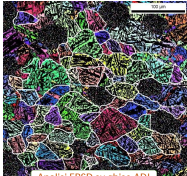
Analisi EBSD su ghise ADI
